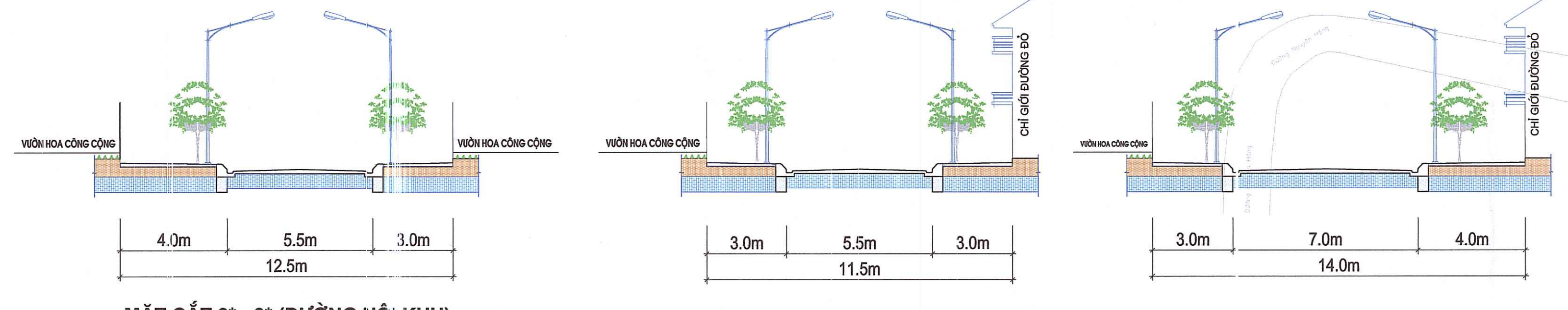
MẶT CẮT 3* - 3* (ĐƯỜNG NỘI KHU)
