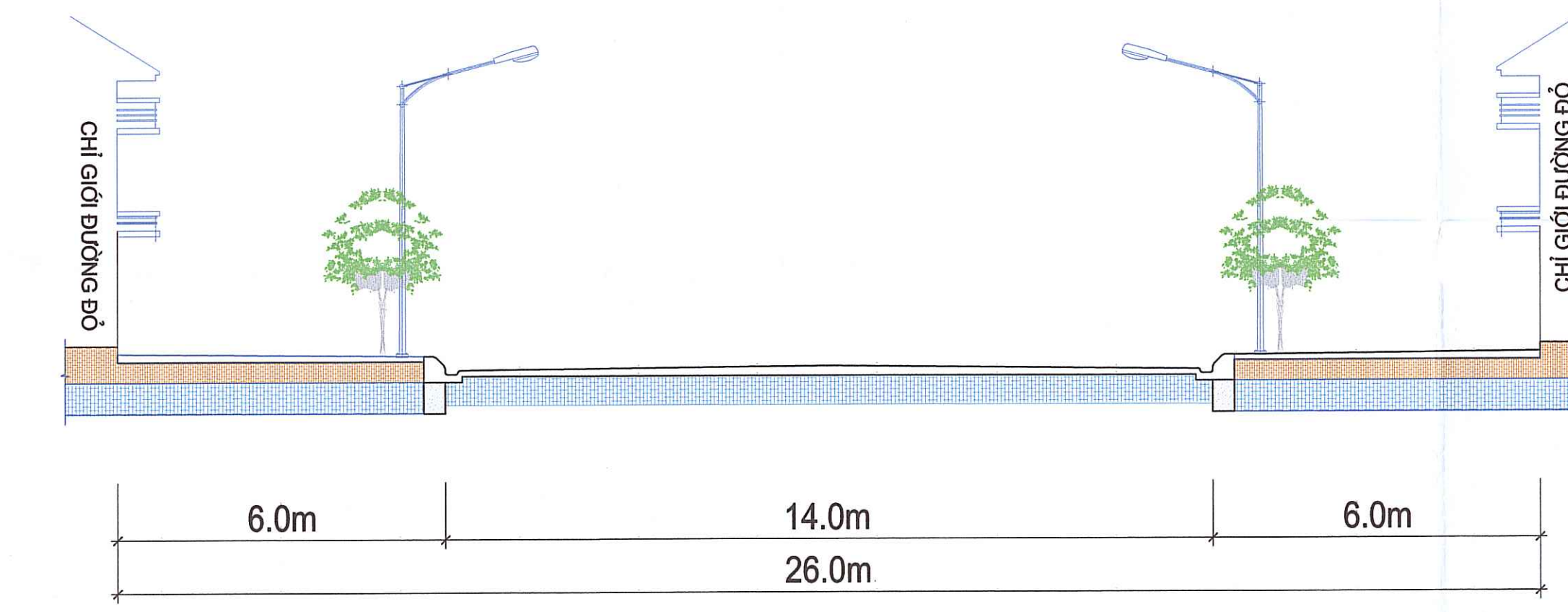
MẶT CẮT 1* - 1* (ĐƯỜNG NỘI KHU)
