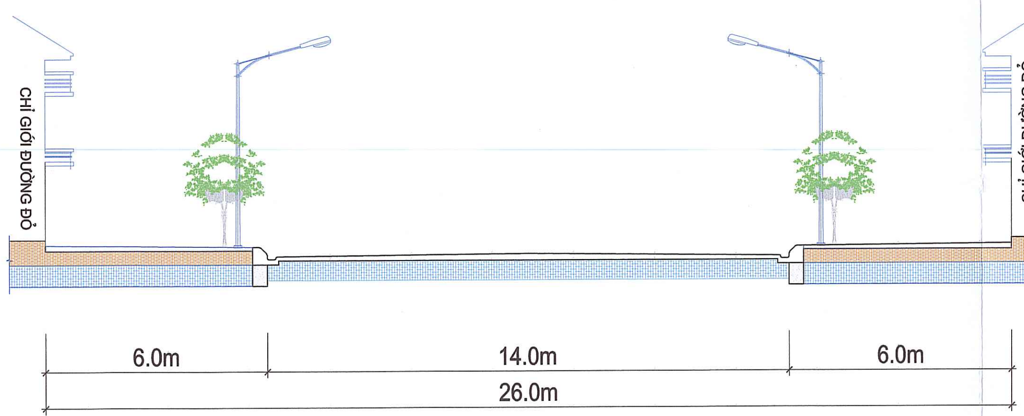
MẶT CẮT 1 - 1 (ĐƯỜNG LIÊN KHU VỰC)
