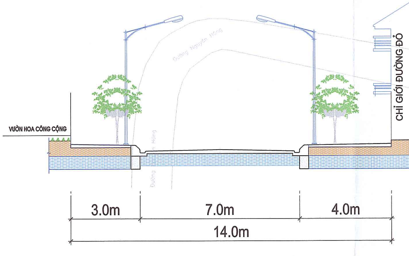
MẶT CẮT 2* - 2* (ĐƯỜNG NỘI KHU)
