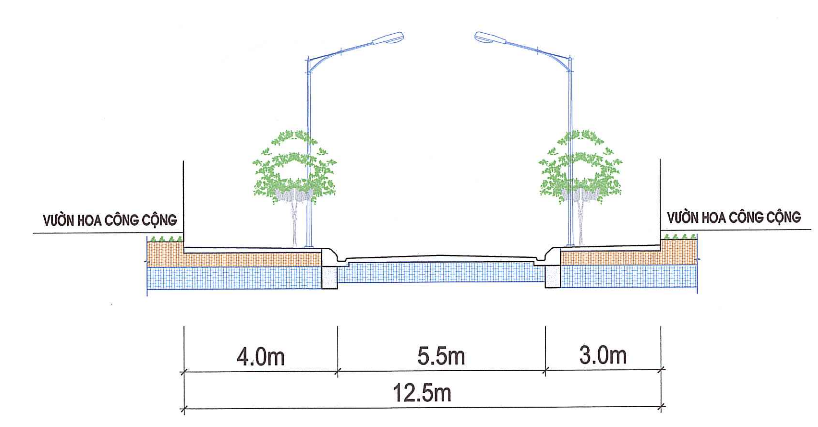
MẶT CẮT 3* - 3* (ĐƯỜNG NỘI KHU)
