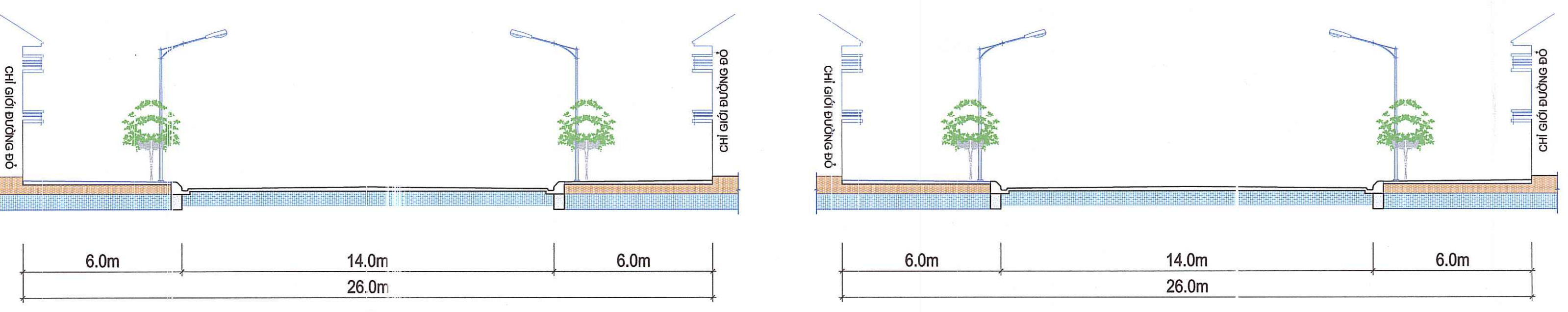
MẶT CẮT 1 - 1 (ĐƯỜNG LIÊN KHU VỰC)
