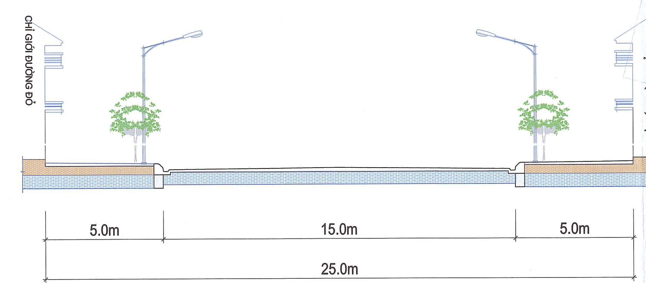
MẶT CẮT 4 - 4 (ĐƯỜNG LIÊN KHU VỰC)
