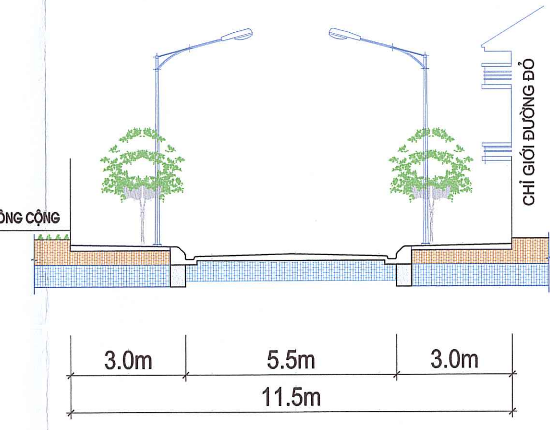
MẶT CẮT 3 - 3 (ĐƯỜNG NỘI KHU)
