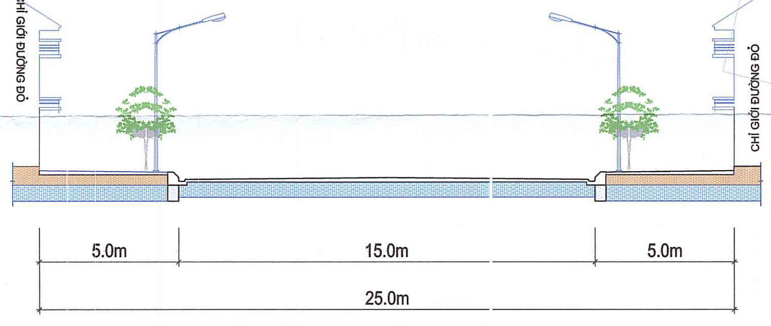
MẶT CẮT 4 - 4 (ĐƯỜNG LIÊN KHU VỰC)
